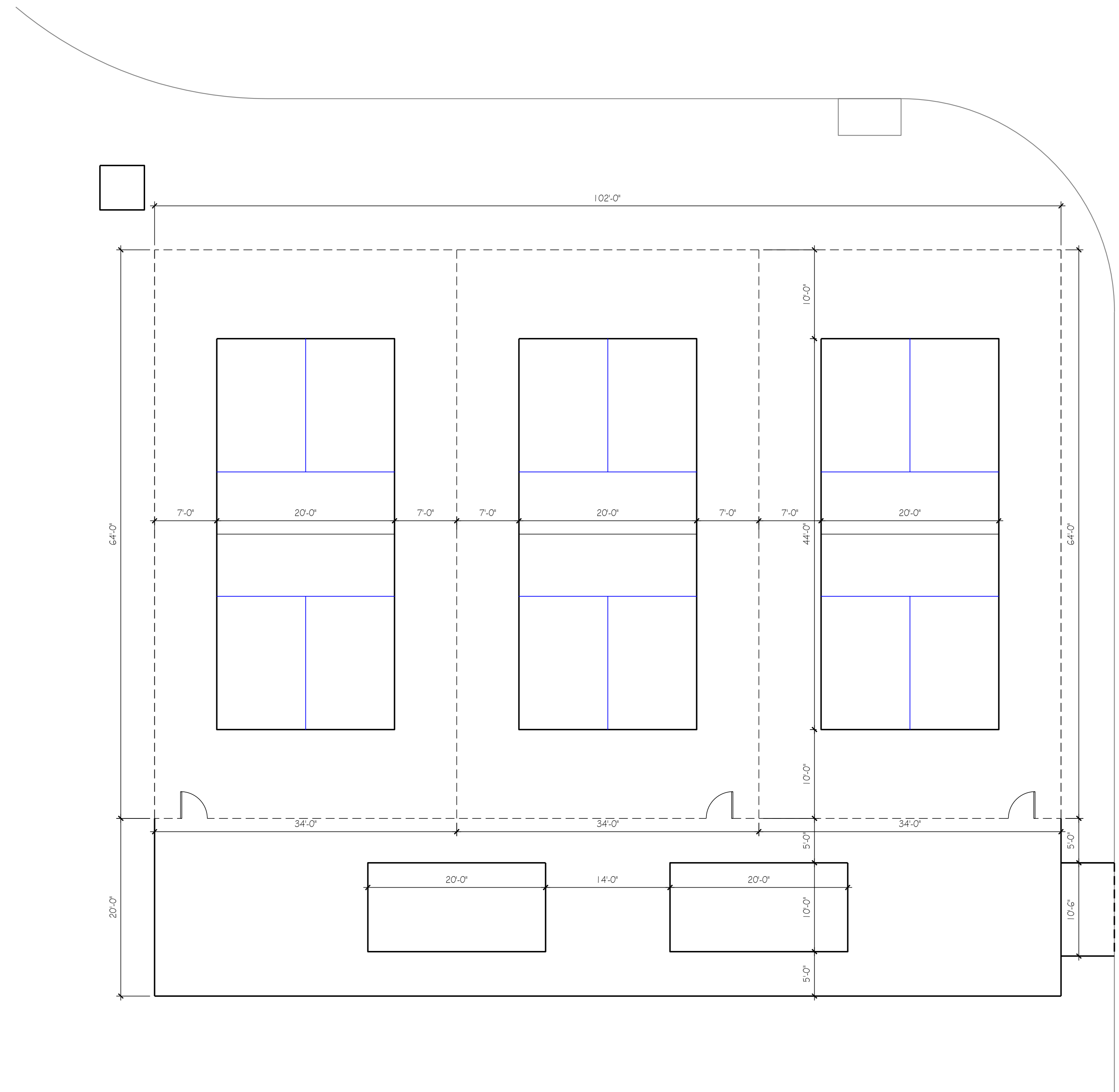
SITEPLAN ① SCALE: 1/8" = 1'-0"
